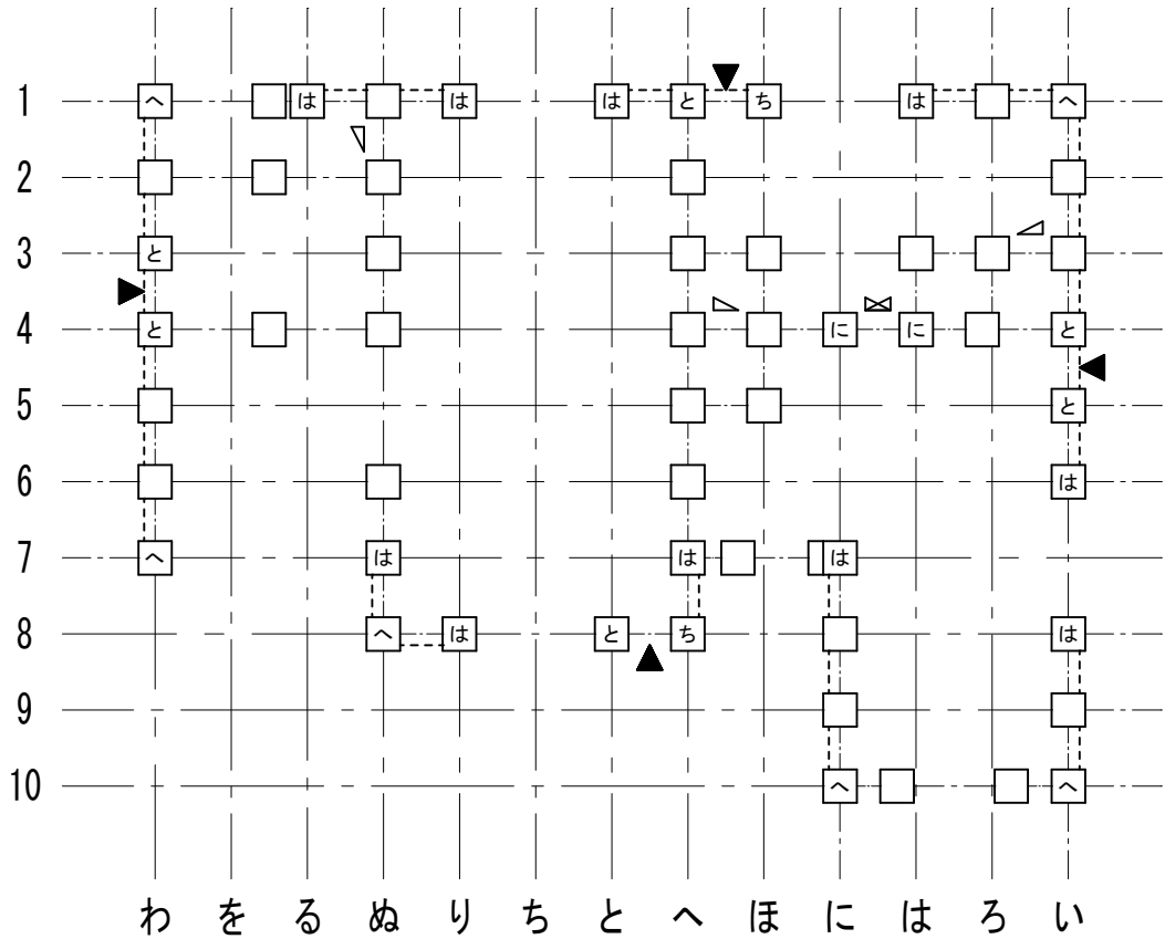
1 階柱壁伏図
